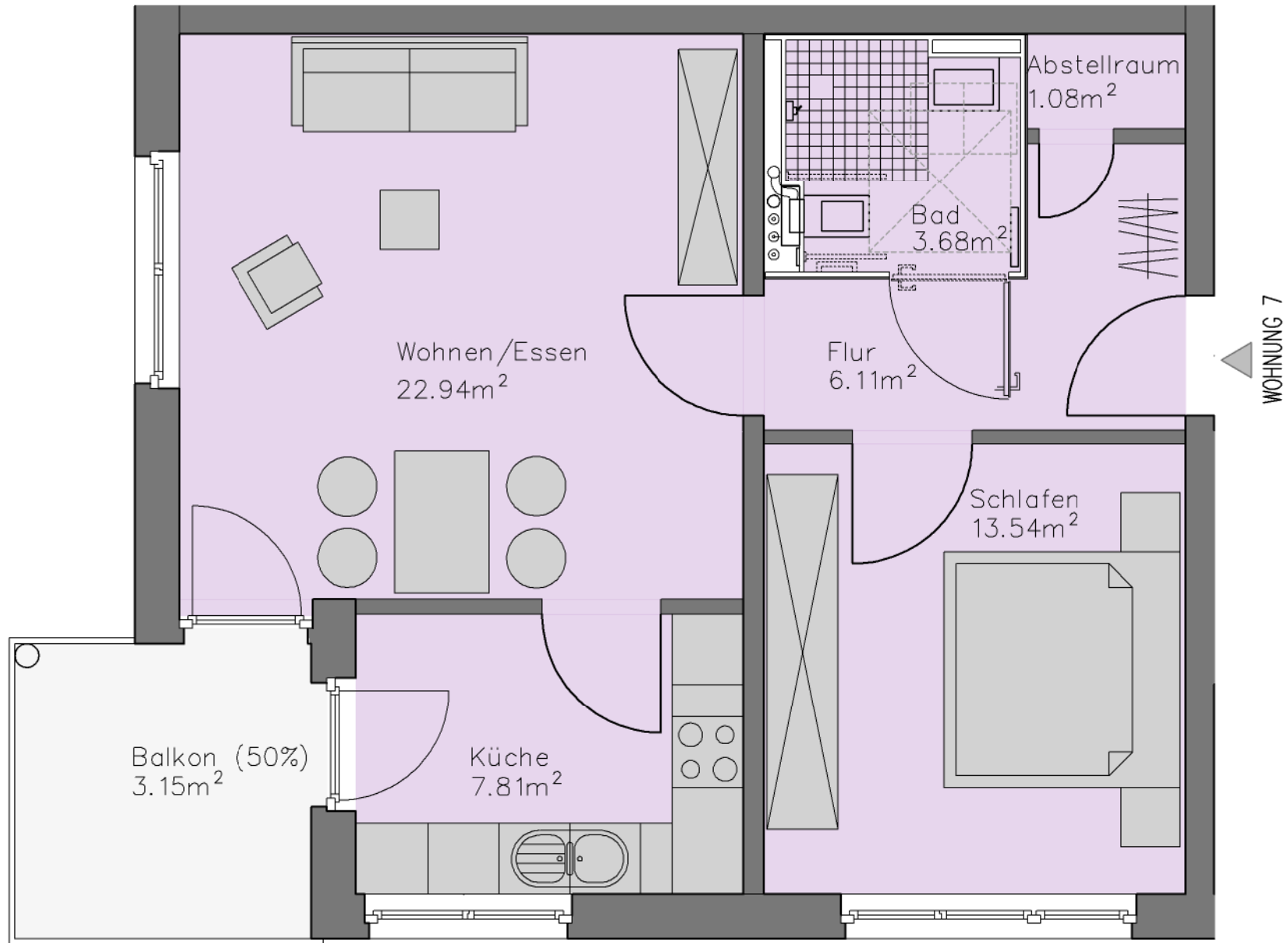
Wohnung 7– 58.31m 2
