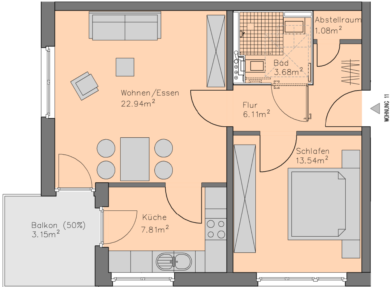
Wohnung 11– 58.31m 2
